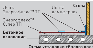
Схема установки тёплого пола
